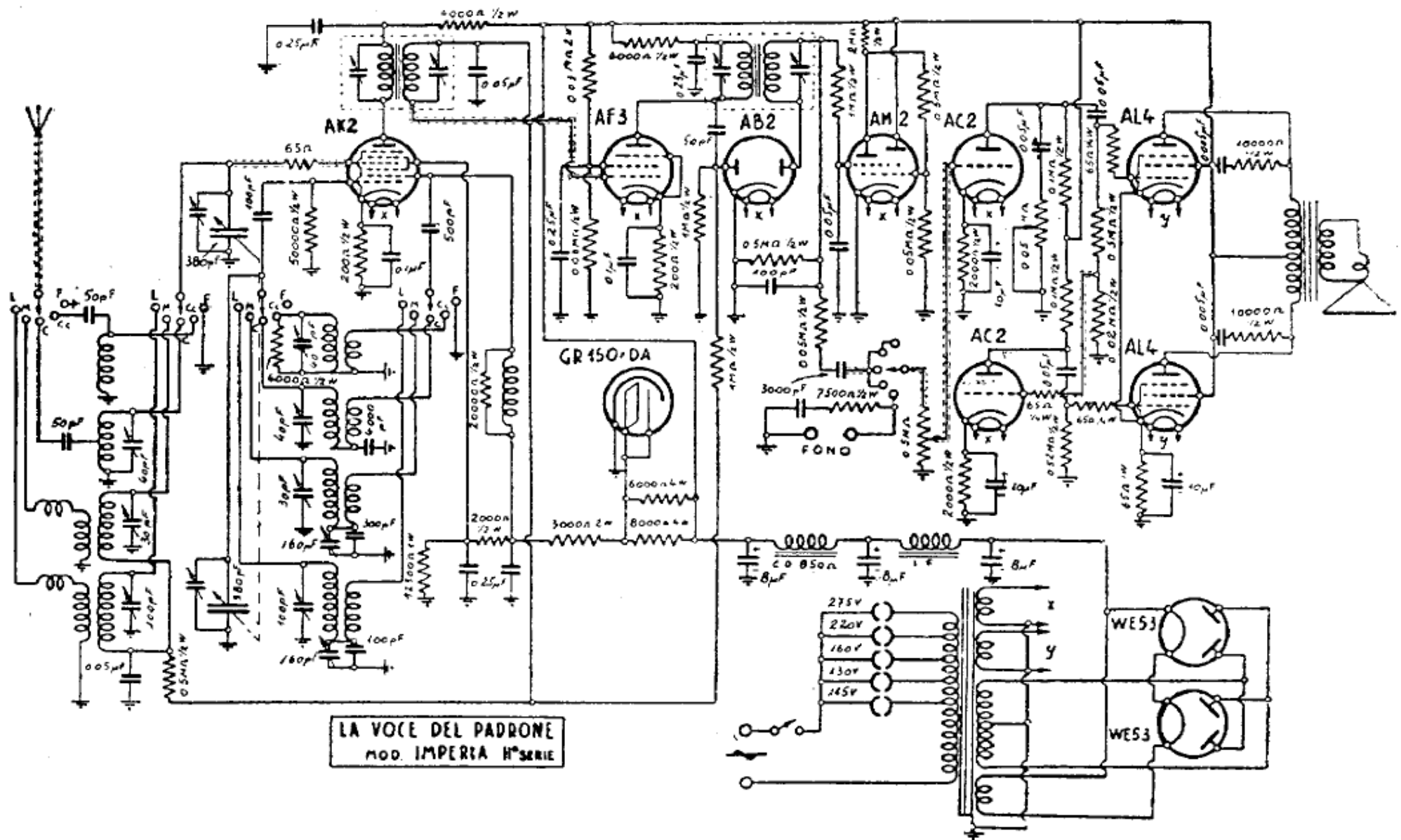
LA VOCE DEL PADRONE. — Mod. « Imperia II serie », - Produzione 1937. - Media frequenza: 465 kHz.
